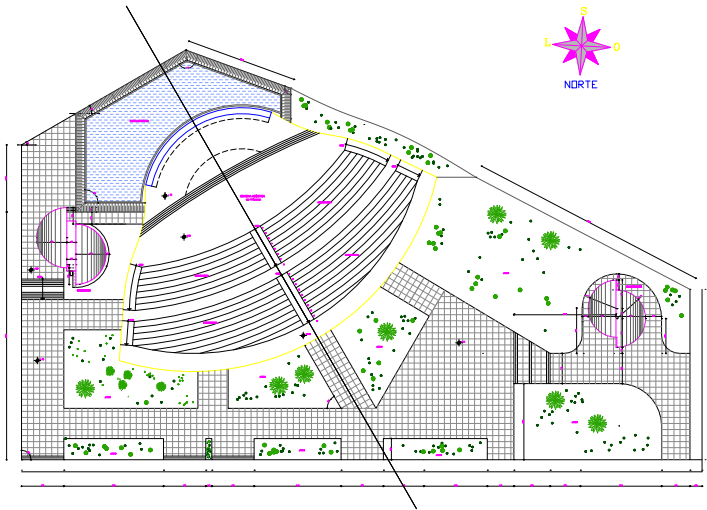
ESCALA 1/100
